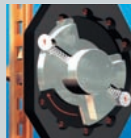
Girando la maniglia i bulloni di sicurezza dotati di molla (1) si Appoggiano con un Klik negli alloggiamenti (2).
