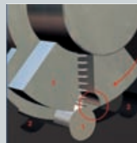
Nel tentativo di intrusione i bulloni di Sicurezza (1) vengono pressati nell'alloggiamento attraverso un secondo elemento accoppiato (3)
